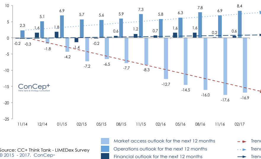
Fig. 3: LIMEDex Sub-Indexes
